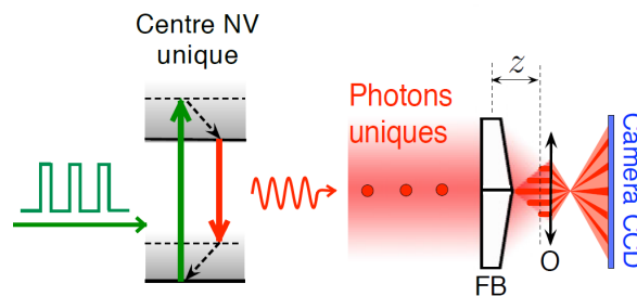
Bi-prisme de Fresnel : enregistrement du champ d’interférences
