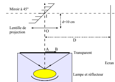
FIGURE 1 – Principe du rétroprojecteur
