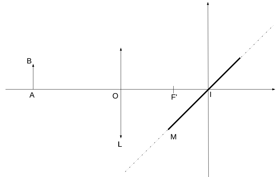
FIGURE 2 – Construction de l'image géométrique
